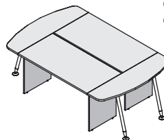
Габариты: 220x143x75
