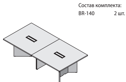
Габариты: 280x140x76
