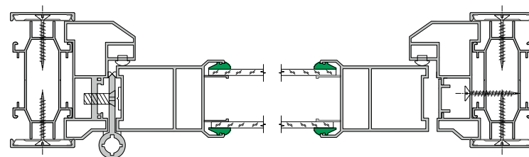
Схема А Перегородка глухая • Заполнение: МДФ, цвет венге.
